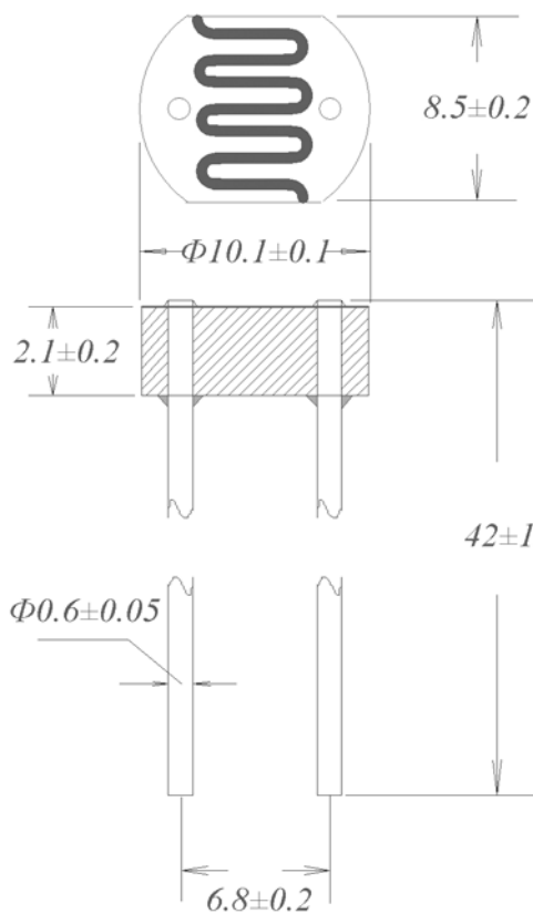
外形尺寸圖 單位：mm
